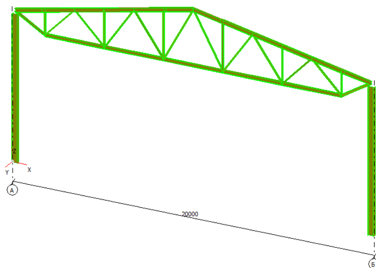
Рис. 1. 9. Рама с ферменным ригелем
