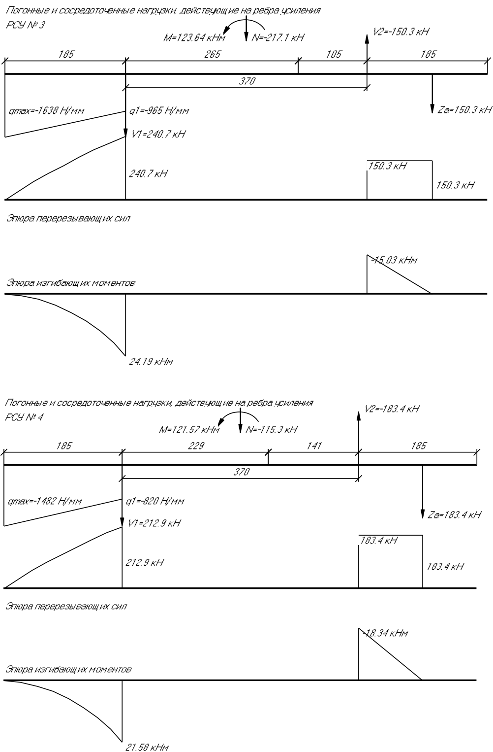
Рис. 2. Расчетная схема для ребра по оси X
